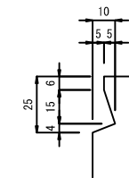
A - A 断面 S=1:2
