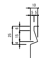
A - A 断面 S=1:2
