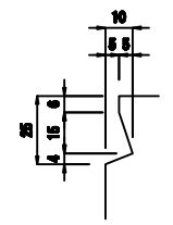
A - A 断面
